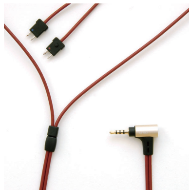
irect_03_b12f_120 2.5 4極プラグ - 2pin(for FitEar)(l/r) 6n+4n 導体ツインリード構造 pvc ジャケット 2.5-4p:金メッキ仕上げ 2pin:ロジウムメッキ仕上げ 長さ:1.2m jan:4534165013101
