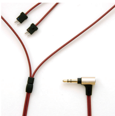
irect_03_ub3f_120 3.5 ステレオプラグ - 2pin(for FitEar)(l/r) 6n+4n 導体ツインリード構造 pvc ジャケット 3.5-3p:金メッキ仕上げ 2pin:ロジウムメッキ仕上げ 長さ:1.2m jan:4534165013095
